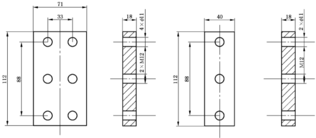
图 B.3 连接板示意图
